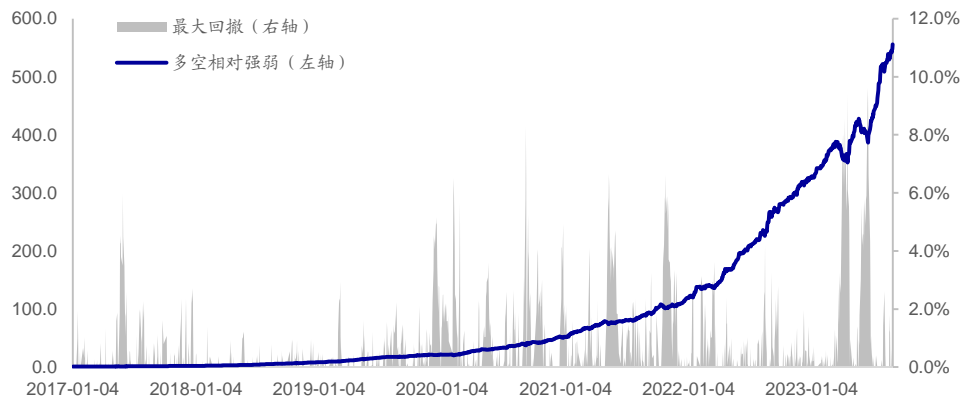
图31 深度学习因子（多颗粒度模型-10日标签）多空相对强弱（2017.01-2023.09）
