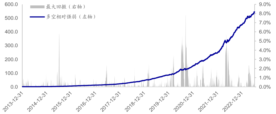
图27 深度学习高频因子(残差注意力 LSTM(48,2)+NN(10))多空相对强弱(2014.01-2023.09)
