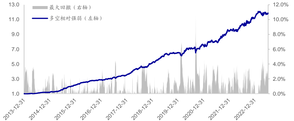
图13 改进反转因子多空相对强弱 (2014.01-2023.09)
