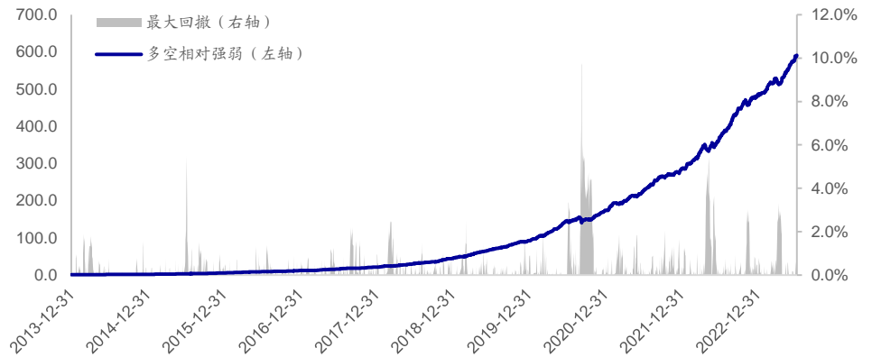
图23 深度学习高频因子 (GRU(50,2)+NN(10)) 多空相对强弱 (2014.01-2023.09)
