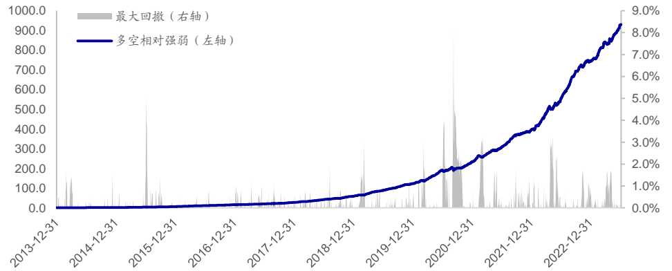
图25 深度学习高频因子（改进 GRU(50,2)+NN(10)）多空相对强弱（2014.01-2023.09）
