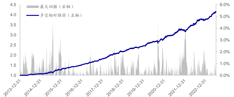
图5 开盘后买入意愿占比因子多空相对强弱（2014.01-2023.10）
