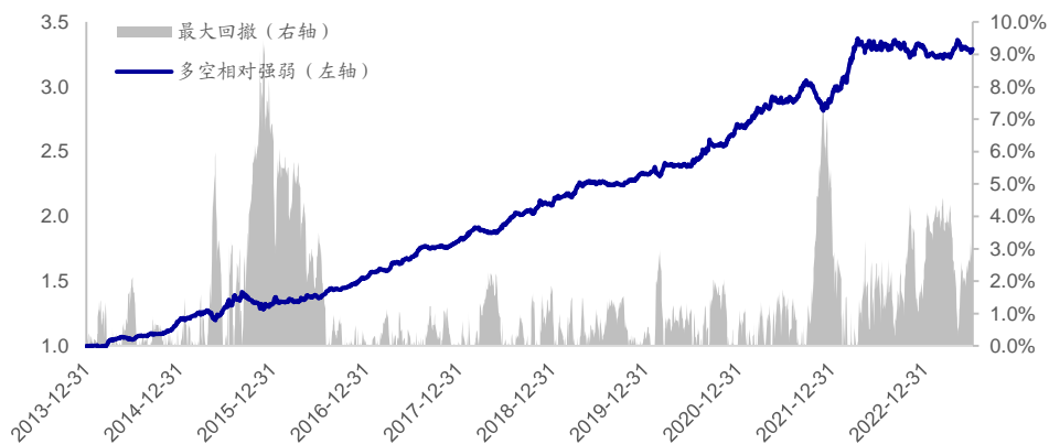
图17 平均单笔流出金额占比因子多空相对强弱 (2014.01-2023.10)
