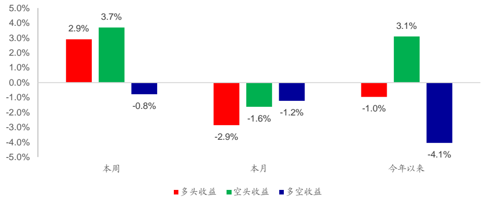
图16 尾盘成交占比多空收益
