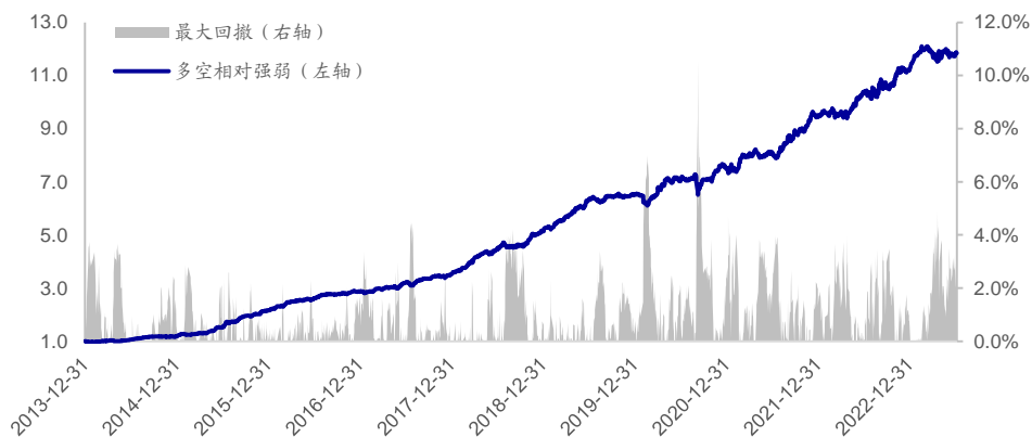
图13 改进反转因子多空相对强弱 (2014.01-2023.10)
