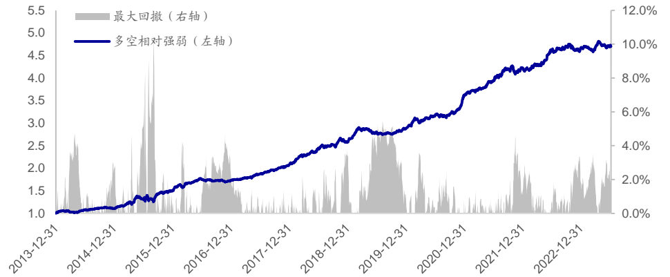
图15 尾盘成交占比因子多空相对强弱 (2014.01-2023.10)
