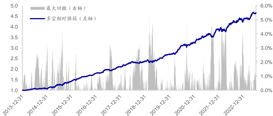
图11 开盘后大单净买入强度因子多空相对强弱 (2014.01-2023.10)
