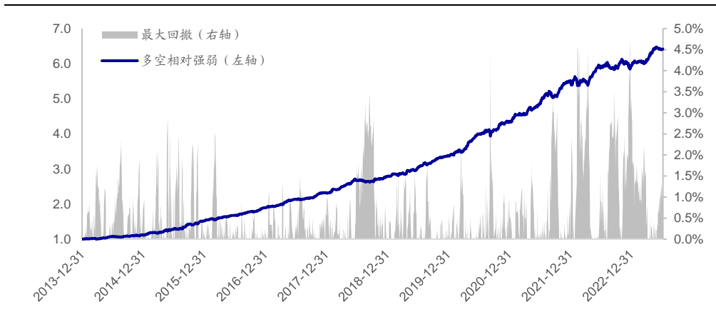
图9 开盘后大单净买入占比因子多空相对强弱 (2014.01-2023.10)
