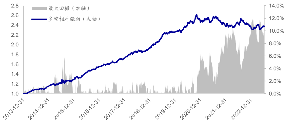
图19 大单推动涨幅因子多空相对强弱 (2014.01-2023.10)
