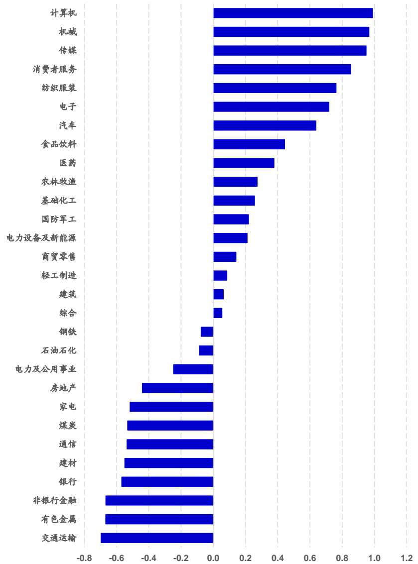
图10 行业拥挤度 (2023.12.15)
