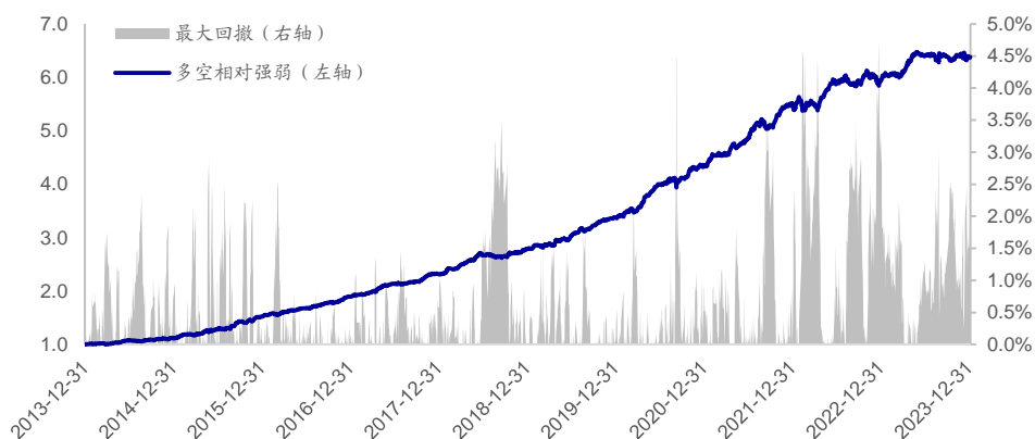
图9 开盘后大单净买入占比因子多空相对强弱 (2014.01-2024.01)
