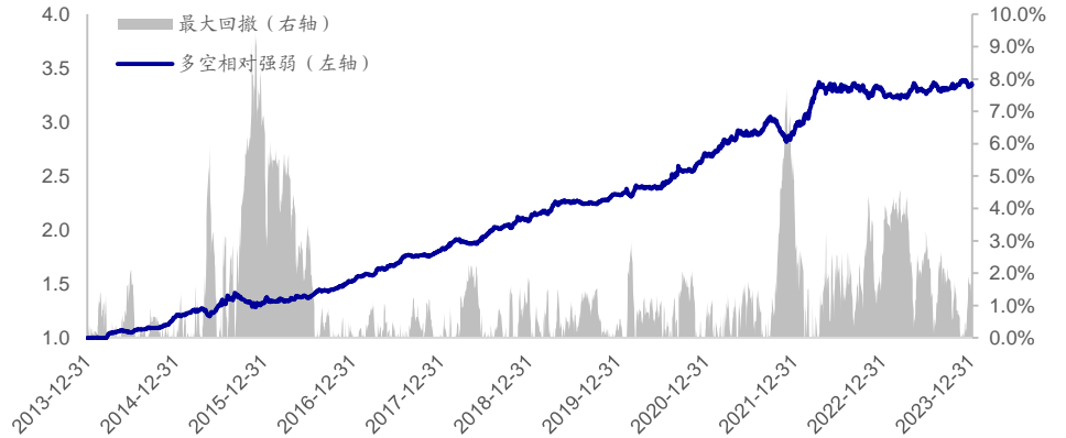
图17 平均单笔流出金额占比因子多空相对强弱 (2014.01-2024.01)
