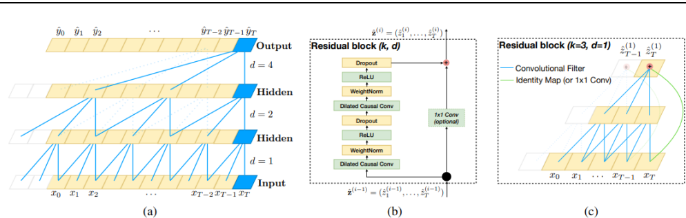
图1 TCN 网络结构示意图
