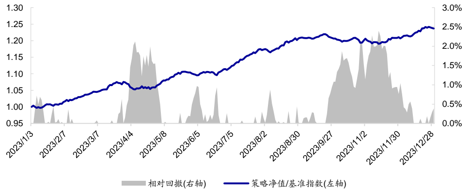
图10 中证 1000AI 增强组合超额净值走势（2023.01-2023.12）
