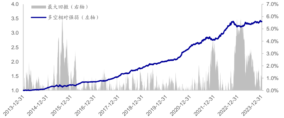
图1 高频偏度因子多空相对强弱 (2014.01-2024.01)
