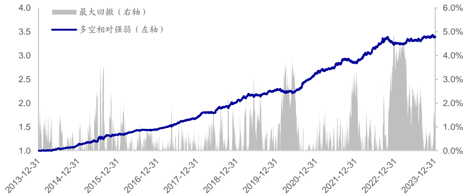
图3 下行波动占比因子多空相对强弱 (2014.01-2024.01)
