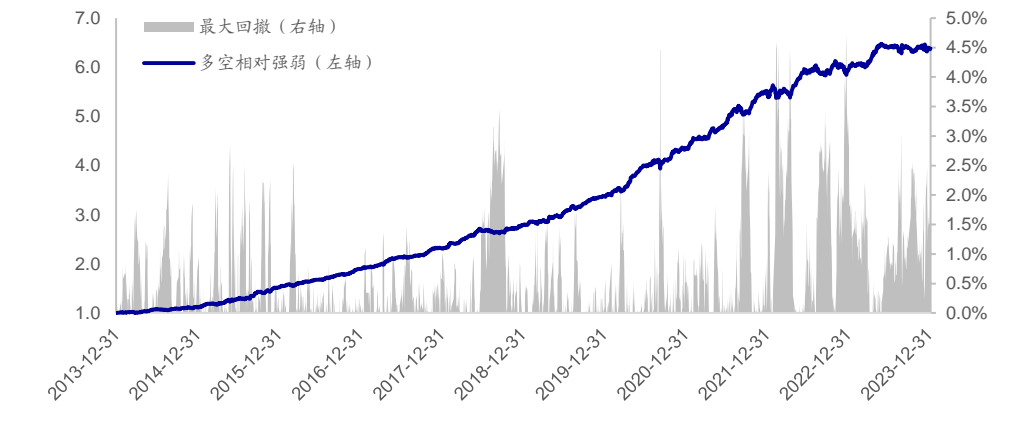
图9 开盘后大单净买入占比因子多空相对强弱 (2014.01-2024.01)
