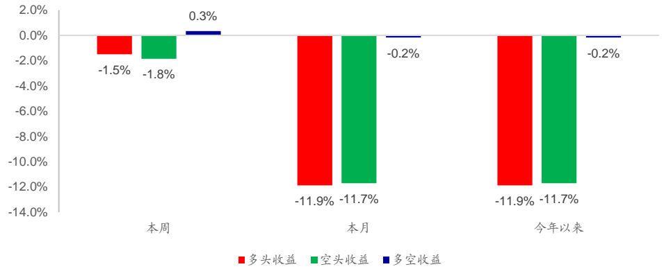
图14 改进反转因子多空收益
