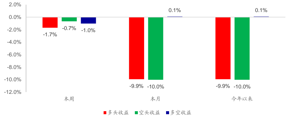
图2 高频偏度因子多空收益
