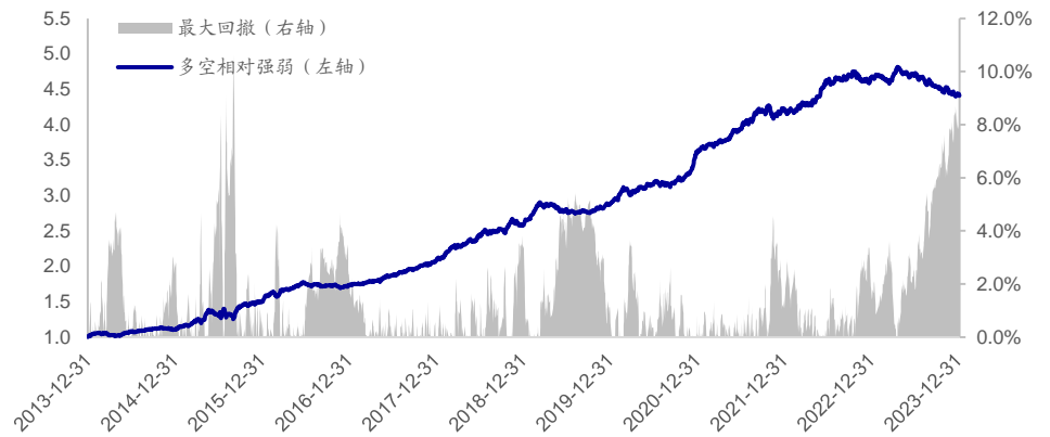
图15 尾盘成交占比因子多空相对强弱（2014.01-2024.01）
