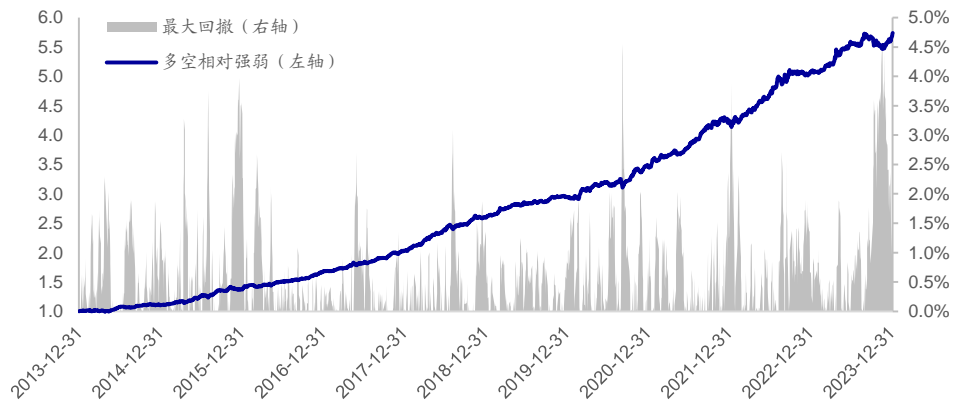
图7 开盘后买入意愿强度因子多空相对强弱（2014.01-2024.01）
