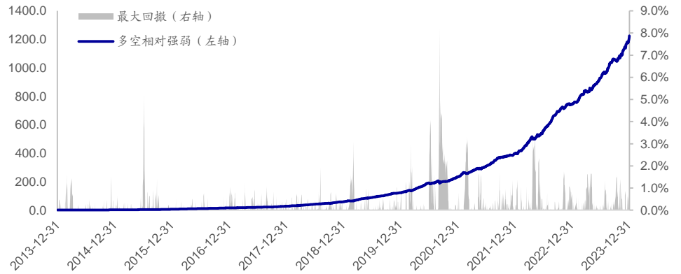
图25 深度学习高频因子（改进 GRU(50,2)+NN(10)）多空相对强弱（2014.01-2024.01）
