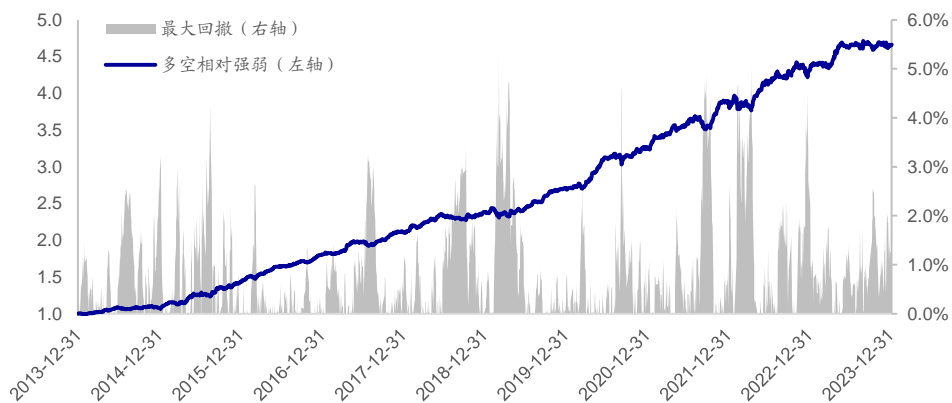
图11 开盘后大单净买入强度因子多空相对强弱 (2014.01-2024.01)
