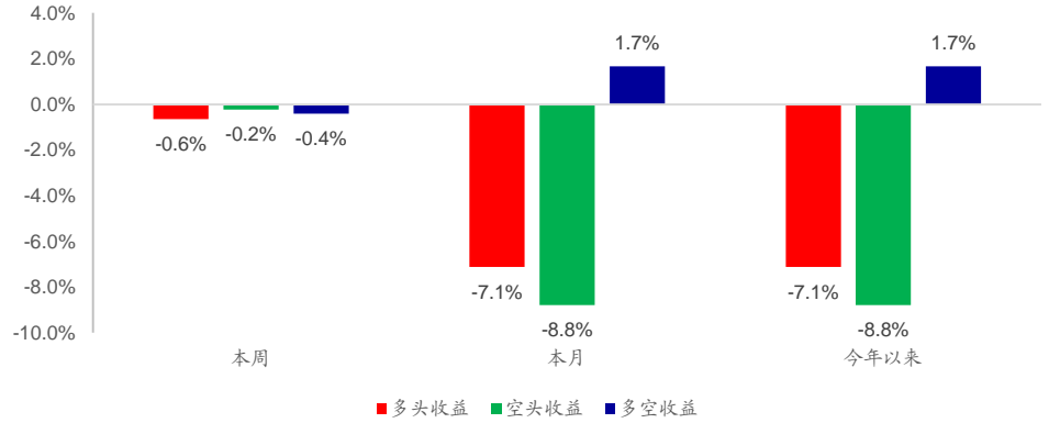
图6 开盘后买入意愿占比因子多空收益
