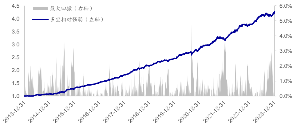
图5 开盘后买入意愿占比因子多空相对强弱（2014.01-2024.01）
