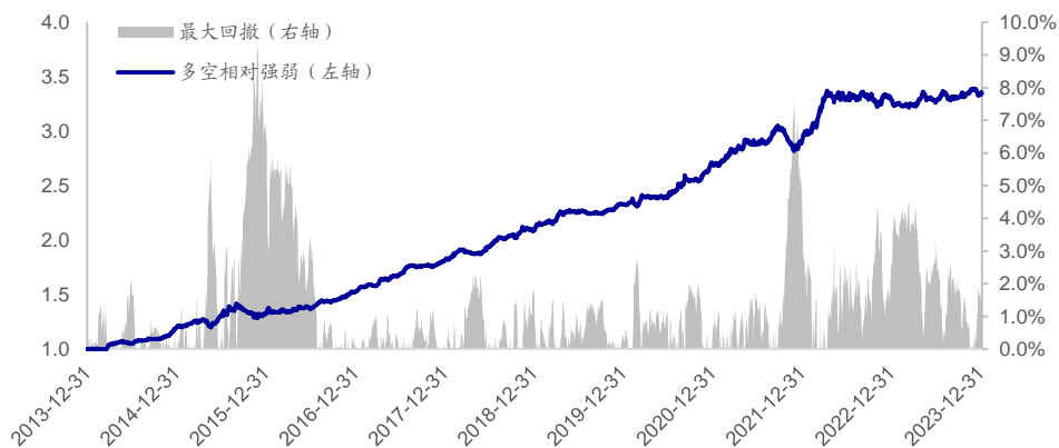
图17 平均单笔流出金额占比因子多空相对强弱 (2014.01-2024.01)
