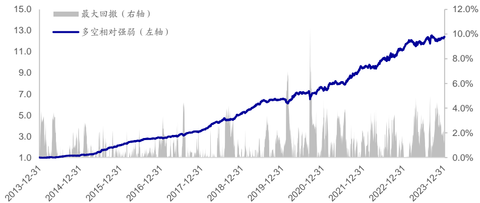
图13 改进反转因子多空相对强弱 (2014.01-2024.01)
