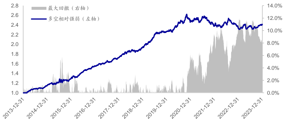
图19 大单推动涨幅因子多空相对强弱 (2014.01-2024.01)
