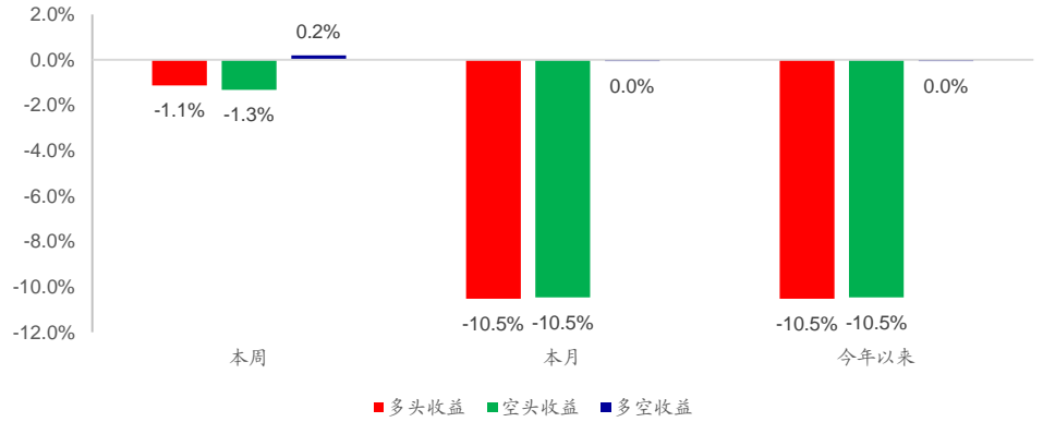
图20 大单推动涨幅因子多空收益
