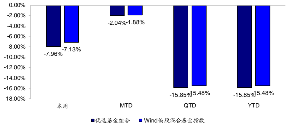
图12 基金优选组合的收益率 (2024.01.02-2024.02.02)
