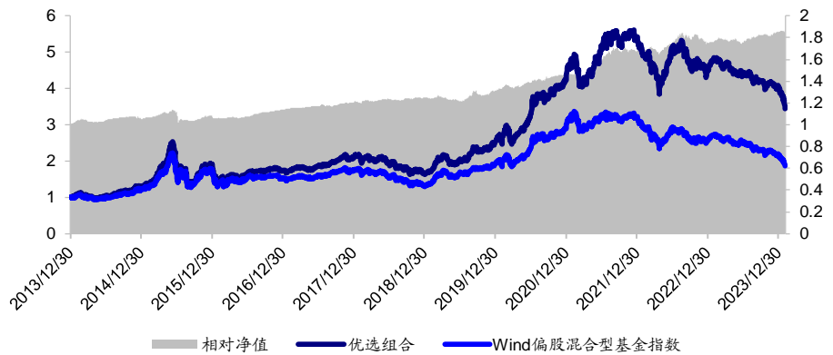
图13 基金优选组合的累计净值 (2014.01.02-2024.02.02)
