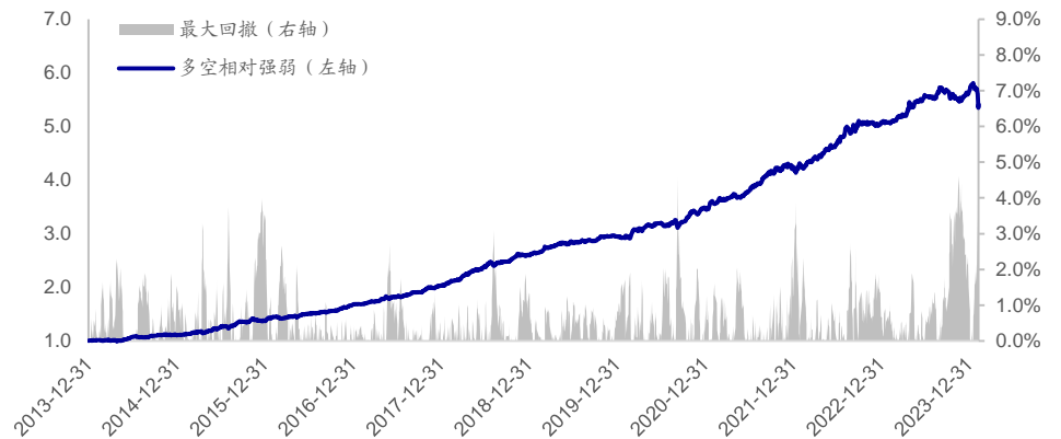
图7 开盘后买入意愿强度因子多空相对强弱（2014.01-2024.03）
