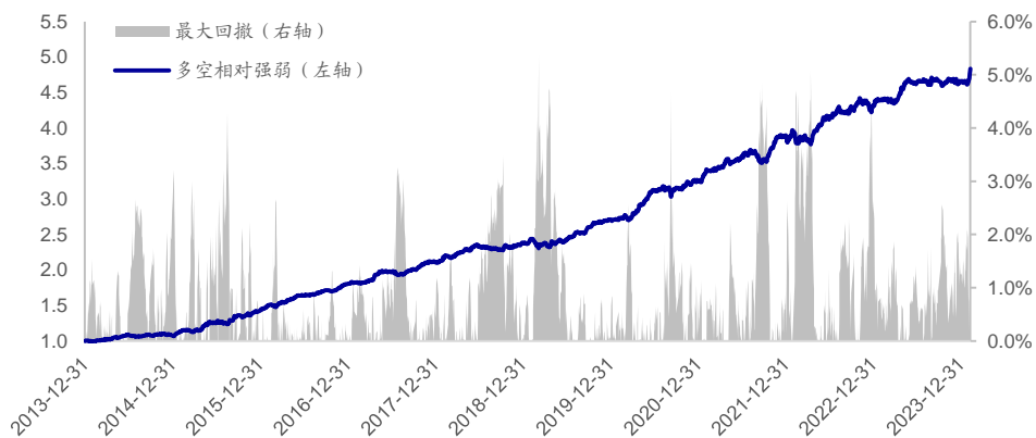
图11 开盘后大单净买入强度因子多空相对强弱 (2014.01-2024.03)
