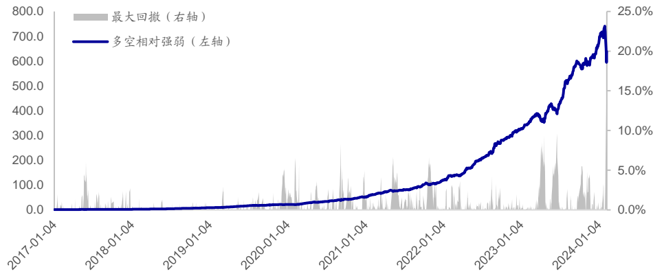
图31 深度学习因子（多颗粒度模型-10日标签）多空相对强弱（2017.01-2024.03）
