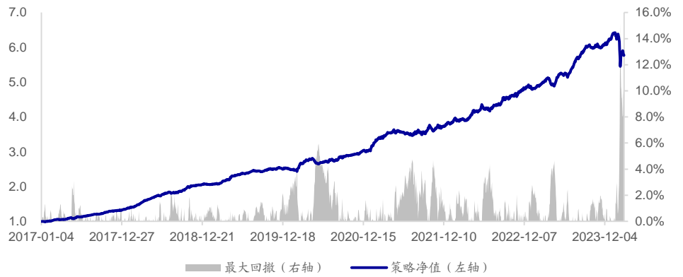
图35 周度调仓的中证 1000 AI 增强组合累计超额收益 (2017.01-2024.03)
