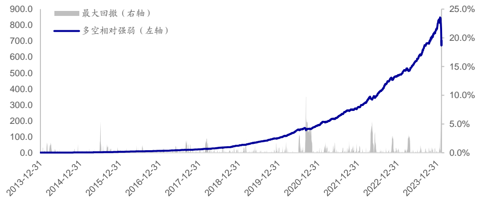
图23 深度学习高频因子 (GRU(50,2)+NN(10)) 多空相对强弱 (2014.01-2024.03)
