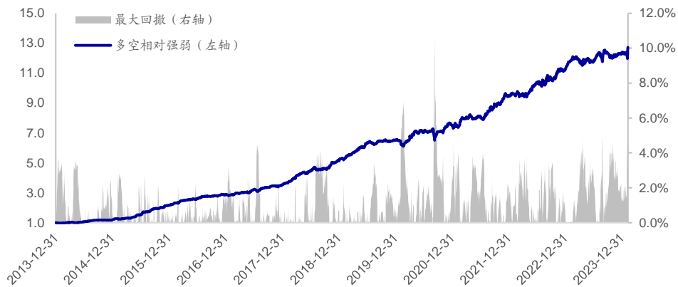
图13 改进反转因子多空相对强弱 (2014.01-2024.03)
