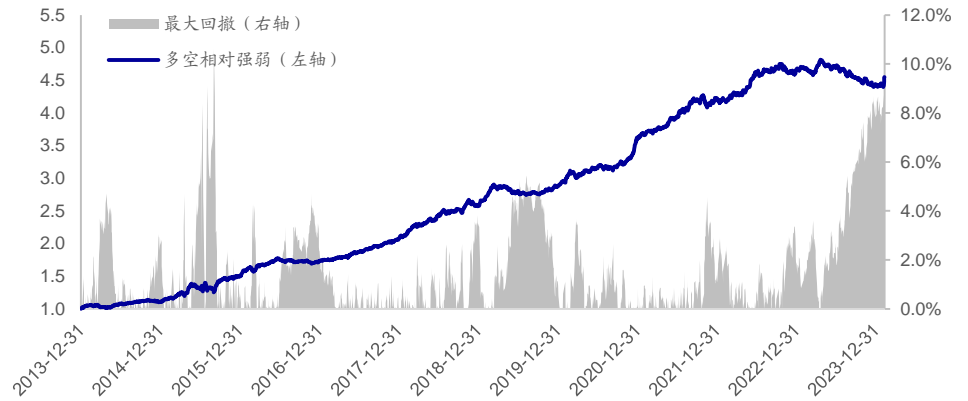
图15 尾盘成交占比因子多空相对强弱 (2014.01-2024.03)
