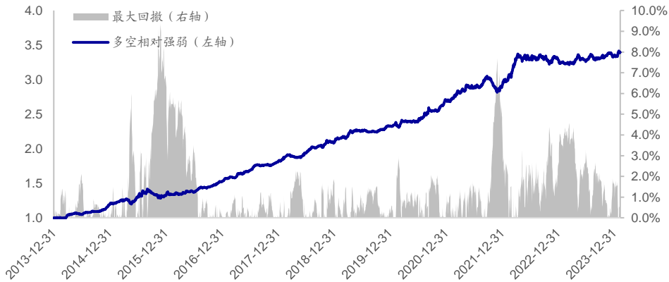
图17 平均单笔流出金额占比因子多空相对强弱 (2014.01-2024.03)
