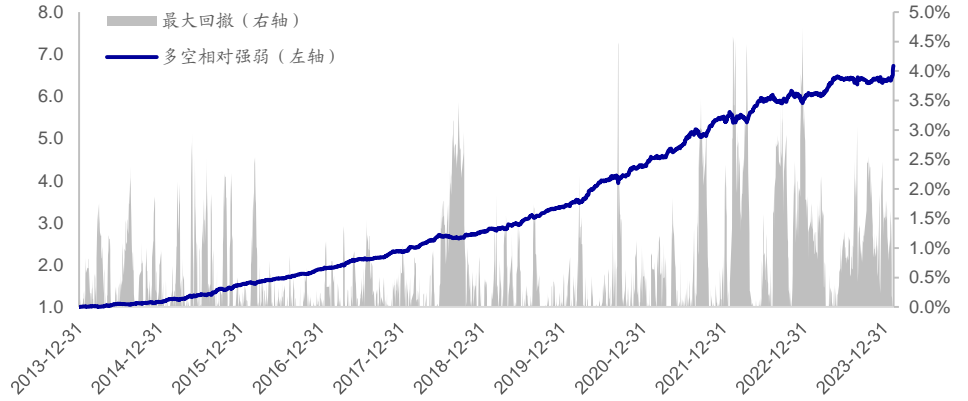
图9 开盘后大单净买入占比因子多空相对强弱 (2014.01-2024.03)
