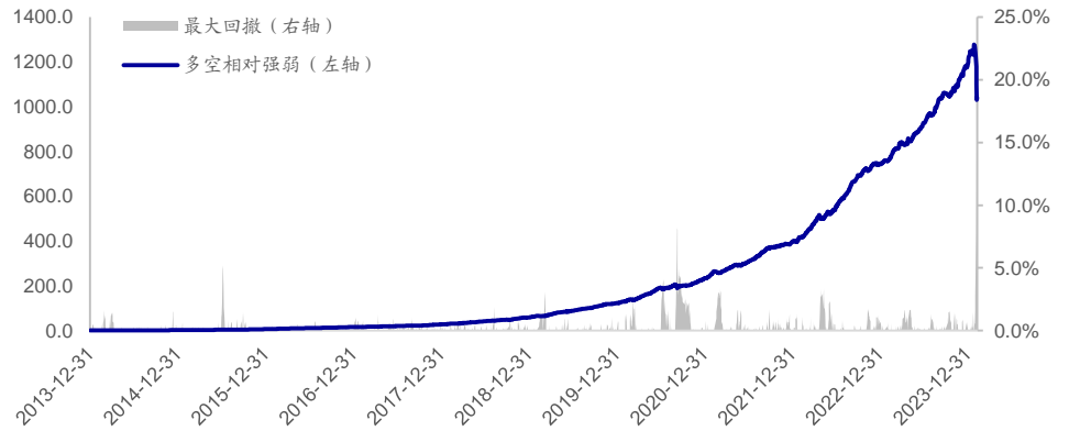
图25 深度学习高频因子（改进 GRU(50,2)+NN(10)）多空相对强弱（2014.01-2024.03）
