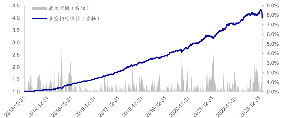
图5 开盘后买入意愿占比因子多空相对强弱（2014.01-2024.03）
