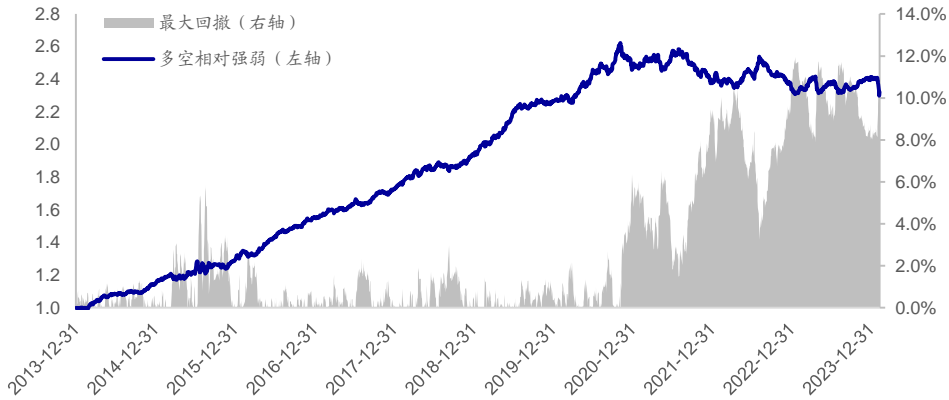
图19 大单推动涨幅因子多空相对强弱 (2014.01-2024.03)
