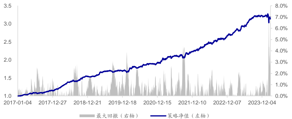
图33 周度调仓的中证 500 AI 增强组合累计超额收益（2017.01-2024.03）
