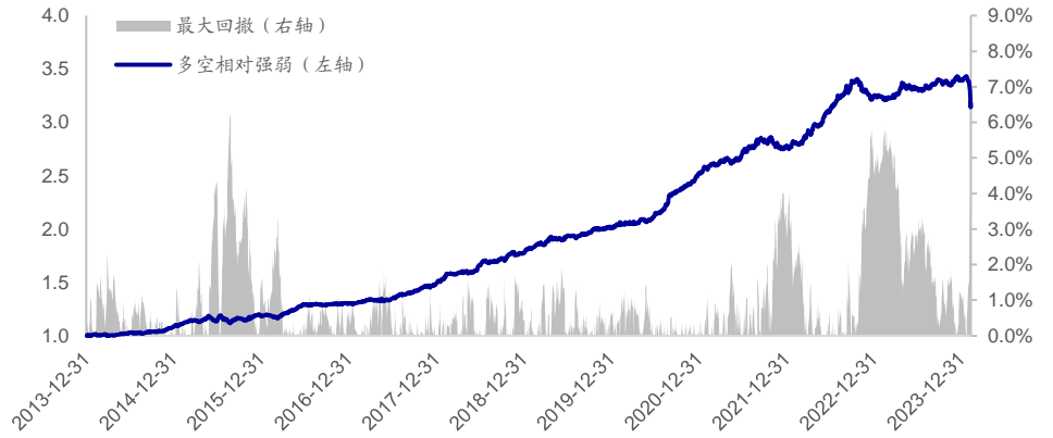
图1 高频偏度因子多空相对强弱 (2014.01-2024.03)
