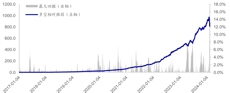
图29 深度学习因子(多颗粒度模型-5日标签)多空相对强弱(2017.01-2024.03)
